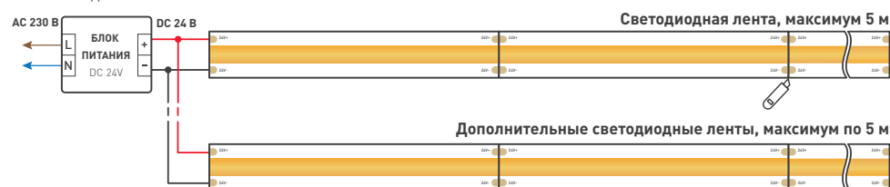
Схема 1. Подключение нескольких светодиодных лент с двух сторон
