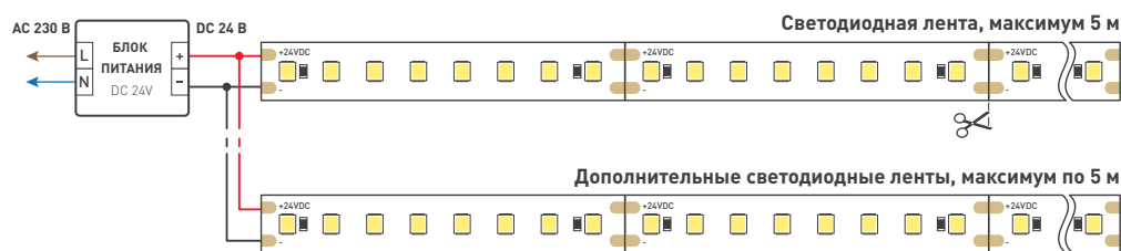
Рис. 1. Подключение нескольких светодиодных лент с одной стороны
