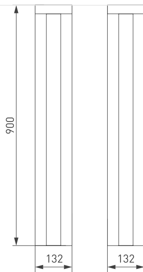
Рис. 1. Чертеж и габаритные размеры
