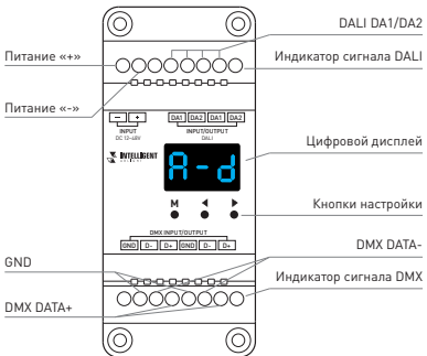
Рис. 3. Схема подключения при конвертации DMX в DALI
