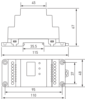
Рис. 1. Габаритный чертеж
