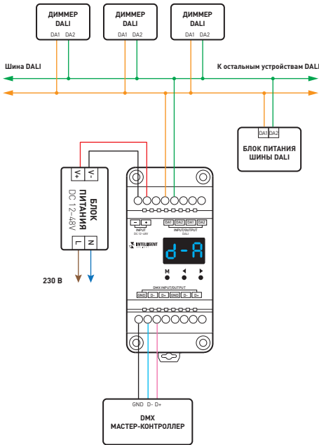
Рис. 3. Схема подключения при конвертации DMX в DALI
