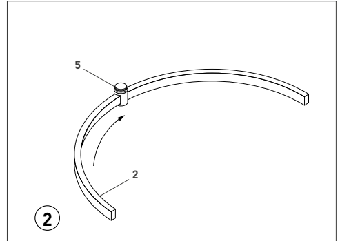
Переместите держатель (5) на середину трека
