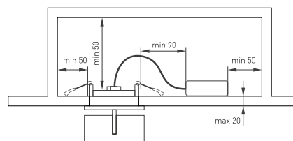
Рис. 3. Установка светильника в нишу
